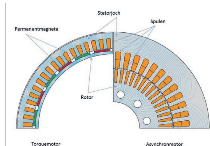
Vergleich Torquemotor (links) und Asynchronmotor: Der Kurzschlussläufer des Rotors im konventionellen Elektromotor (rechts) wird im Torquemotor (links) durch Permanentmagnete (grün/rot) ersetzt.
