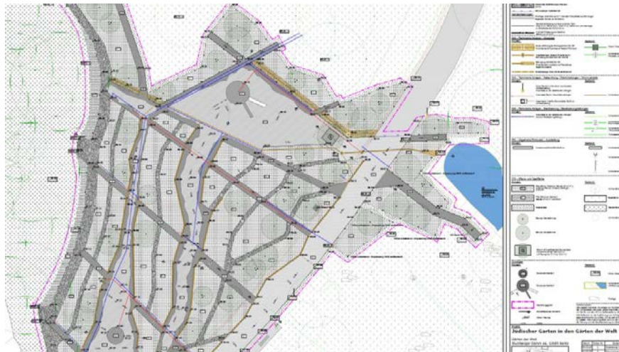
Ausführungsplanung: Technischer Lageplan (Ausschnitt)
