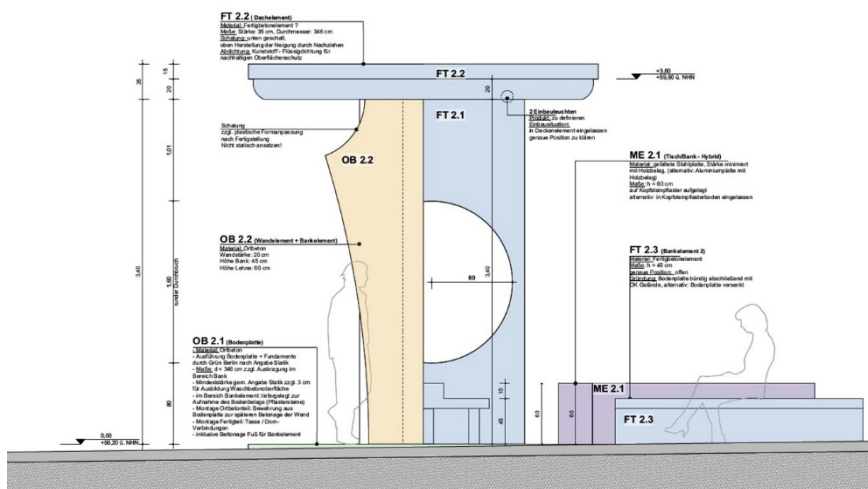
Ausführungsplanung: Vertikalschnitt Skulpturales Gebilde 2
