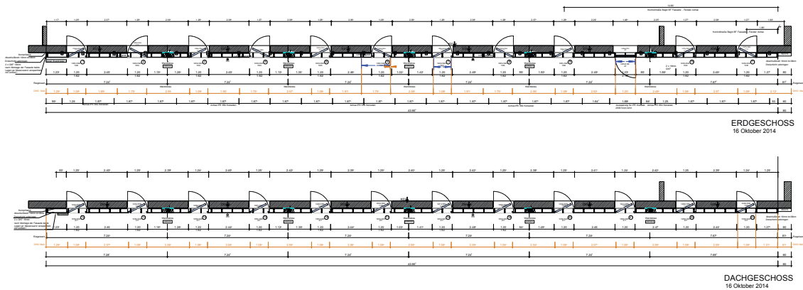
Abb. 31 Horizontalschnitte Holzständerelemente (Zeichnung: BAUFRITZ)
