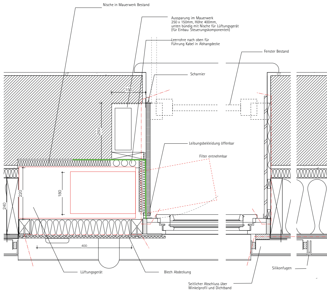
Abb. 14 Horizontalschnitt Fenster
